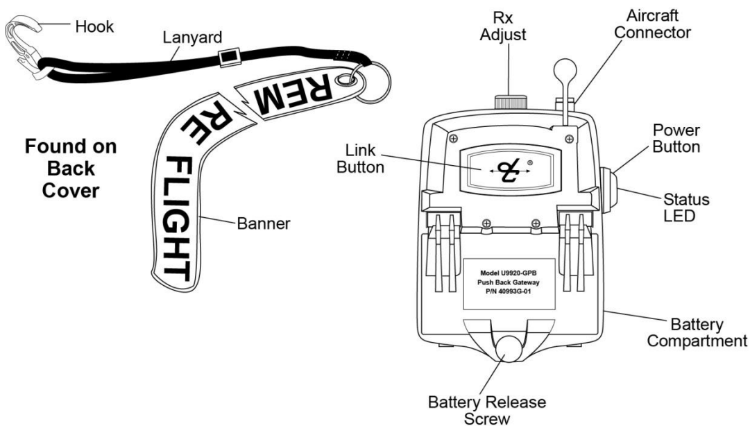
Figure 1 : Vue d'ensemble d'une station individuelle pour opérations de refoulement
